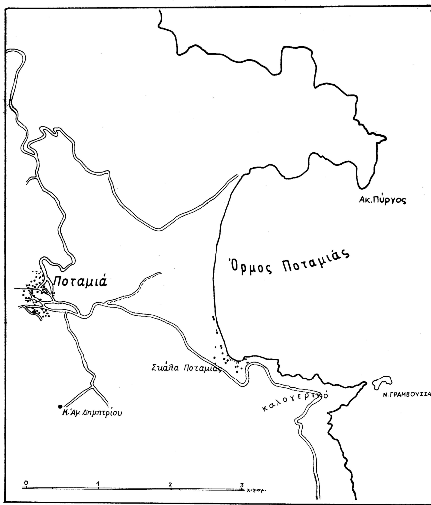
Σχ. 2. Χάρτης της περιοχής Ποταμιάς Θάσου.
